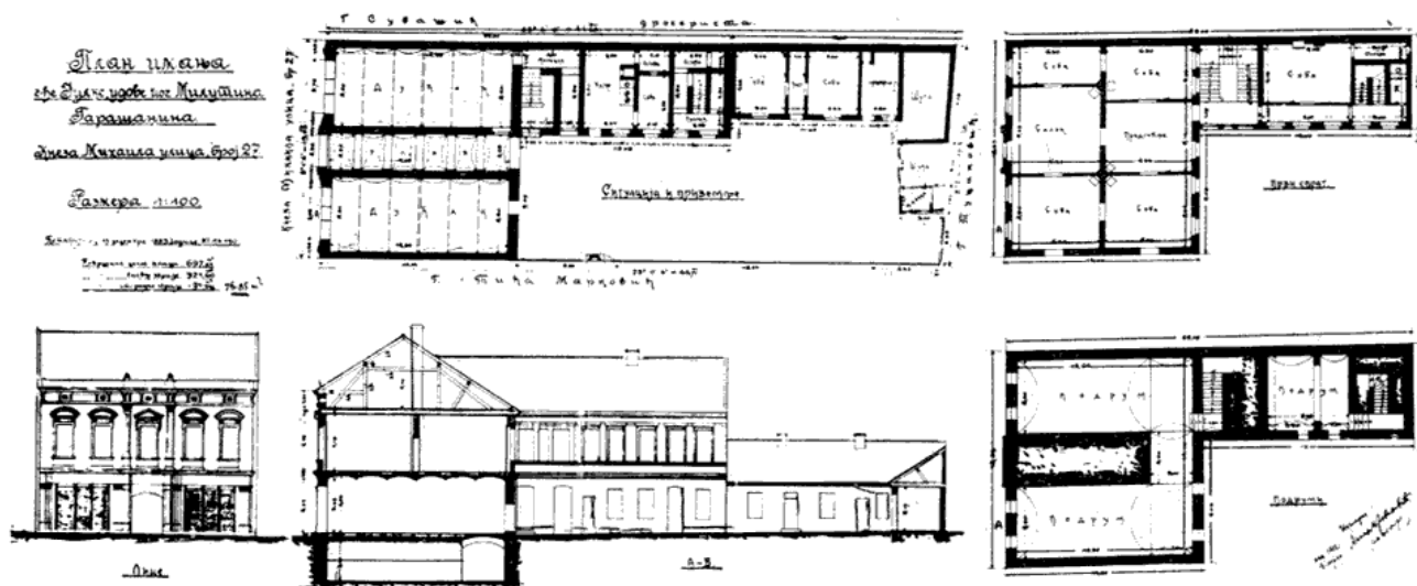
Сл. 12. План стамбене зграде са локалима у Кнез Михаиловој улици бр. 27. Архитектонски снимци 1908. г. инж. Милан М. Јовановић. (МГБ, Ур. 6217).
