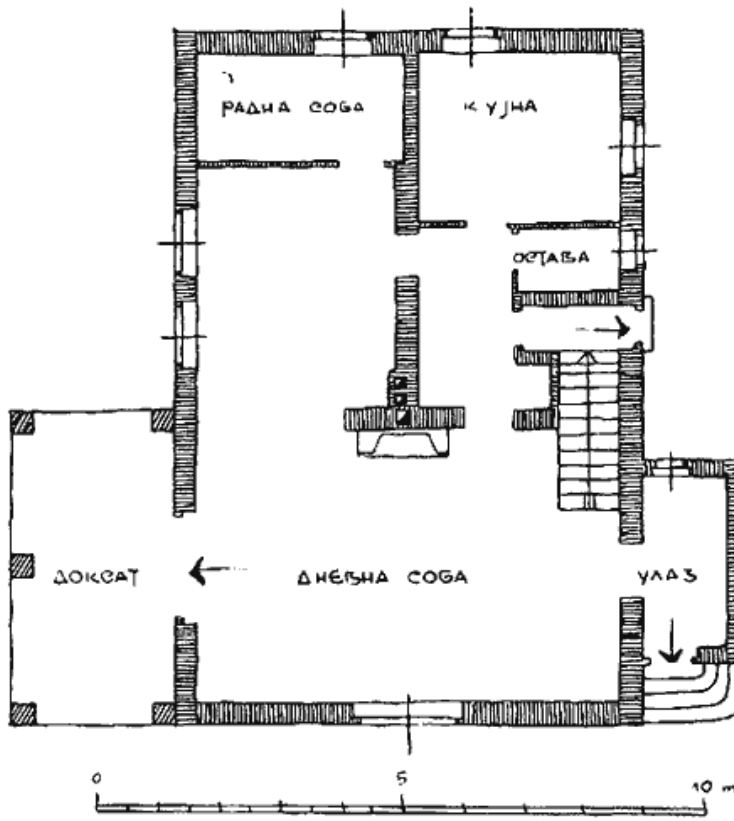
Сл. 5 — Основа приземља.
