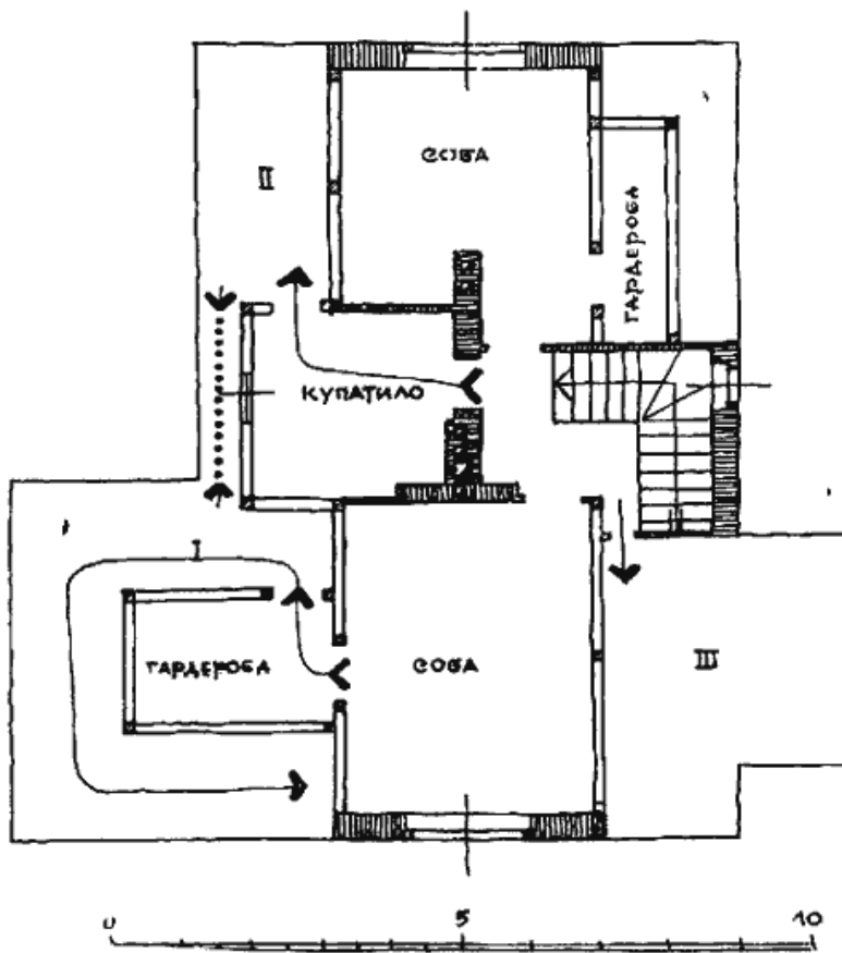
Сл. 6 — Основа мансарде и поткровља.
