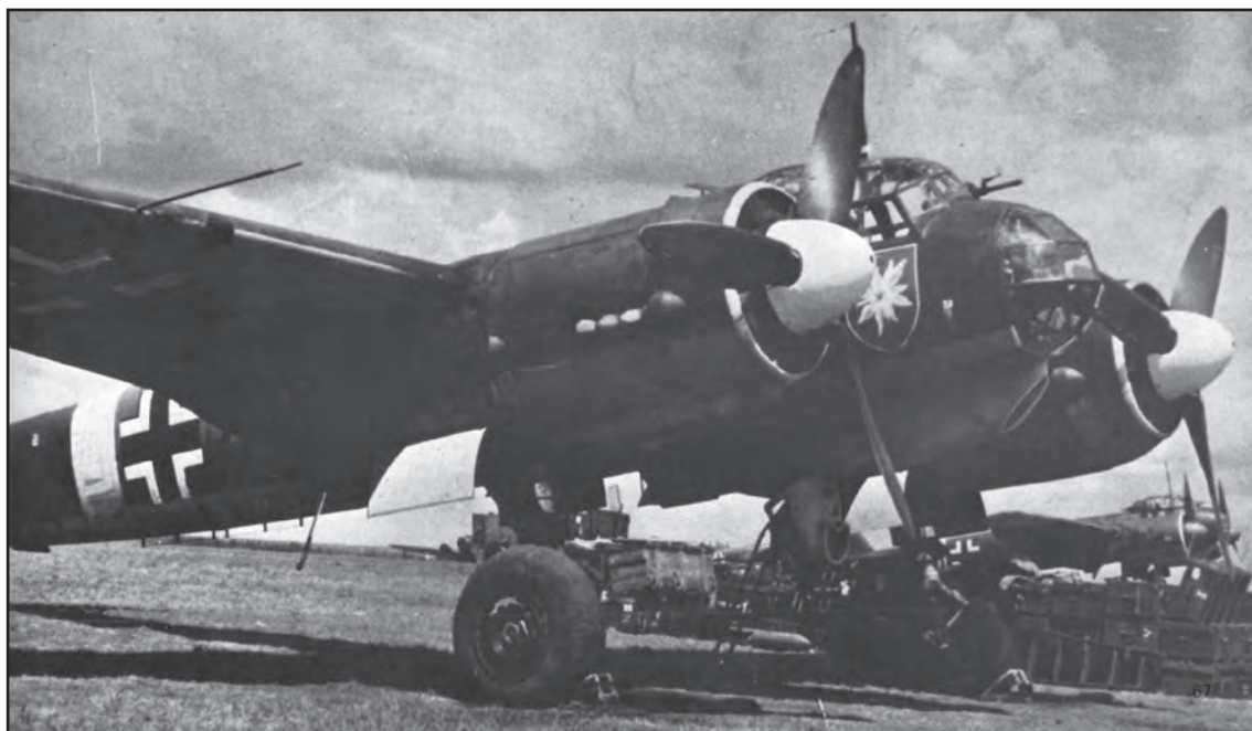
Сл. 5. Бомбардер Јункерс (Ју-88А) из састава дивизије KG-51 „Еделвајс“. Знак јединице је уцртан на боку трупа. Брзина 470 km на сат, долет 2.730 km, носивост 2.500 kg бомби Fig. 5 Bomber Junkers (Ju-88A) from KG-51 airforce division “Edelweiss”. The emblem of the unit is shown on the side of the fuselage. Speed 470 km/h, range 2,730 km, capacity 2,500 kg of bombs
