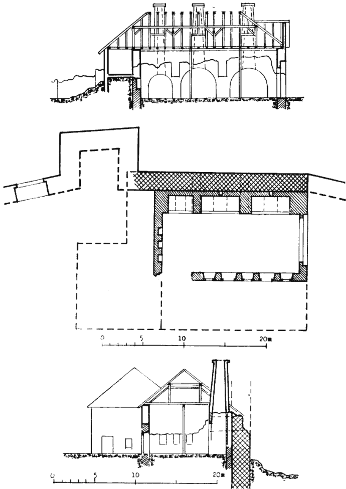
Сл. 7 — Тополивница Првог српског устанка у Доњем Граду у Београду — основа и пресеци
